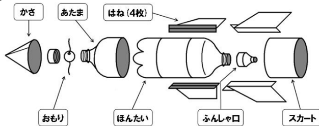
ペットボトルロケットの構造
